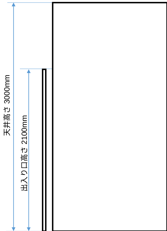
断面横
