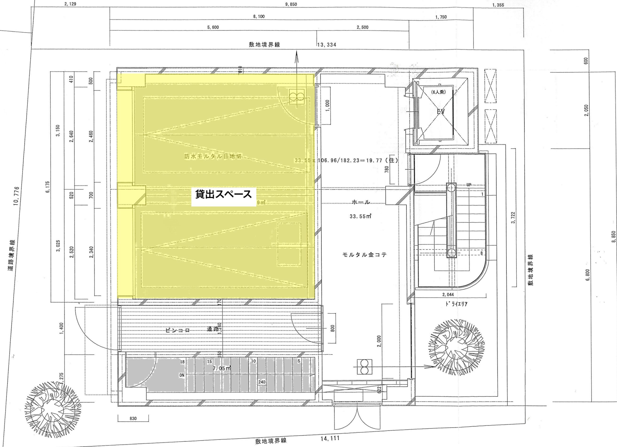
配置図・1階平面図 1/50
